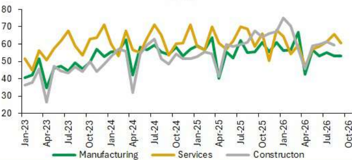
PMI
